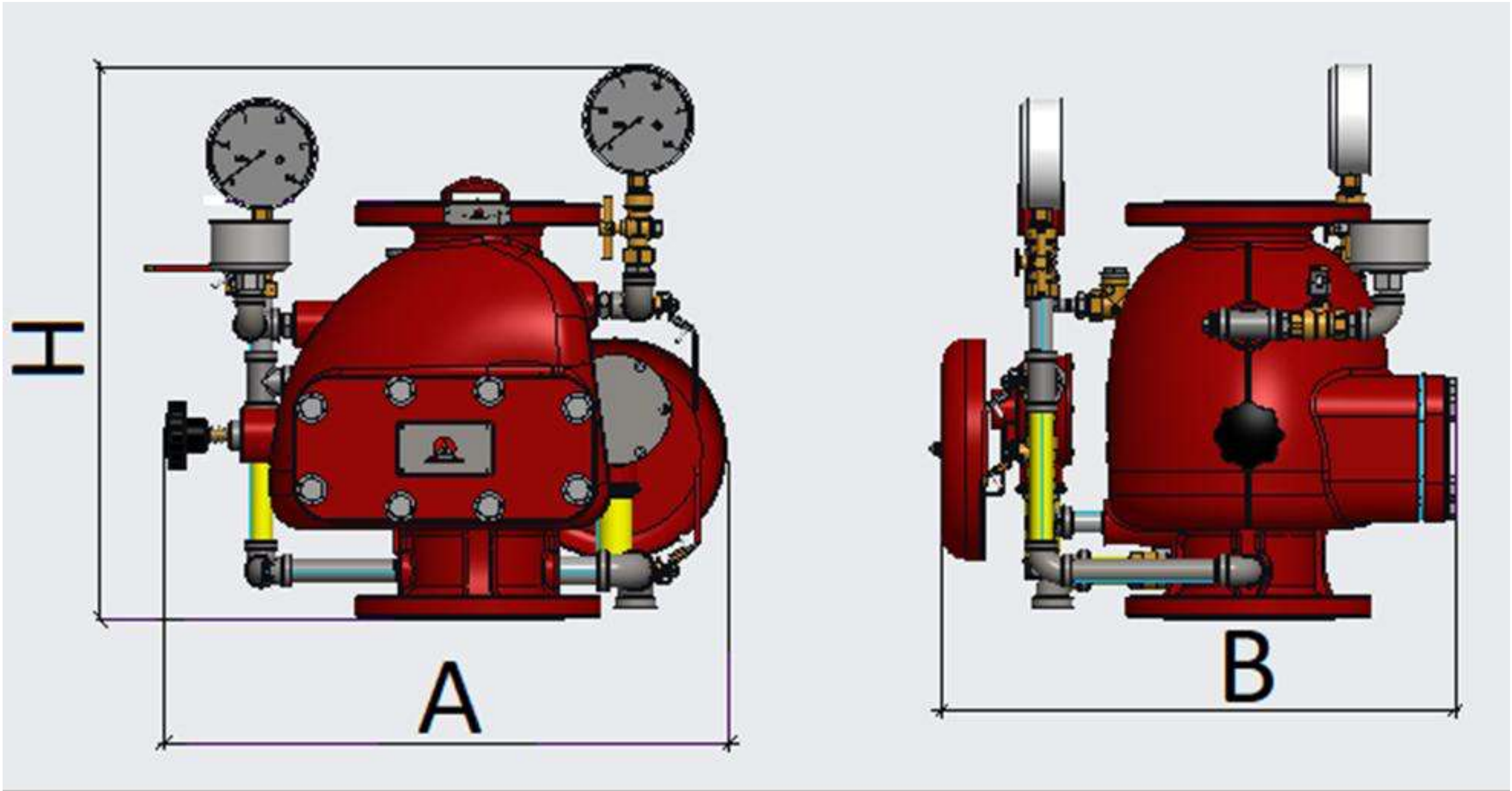
Рисунок 4. Габаритные размеры УУ
